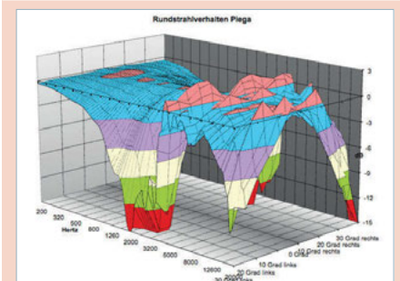
Die Einbrüche im Mitteltonbereich unter größeren Winkeln fallen breitbandig aus, seitliche Hörplätze könnten unter mangelnder Sprachverständlichkeit leiden.
